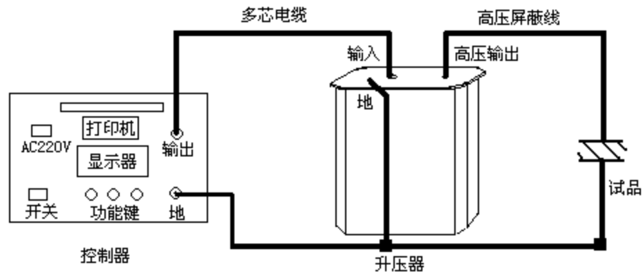
图 4 (连线图)
