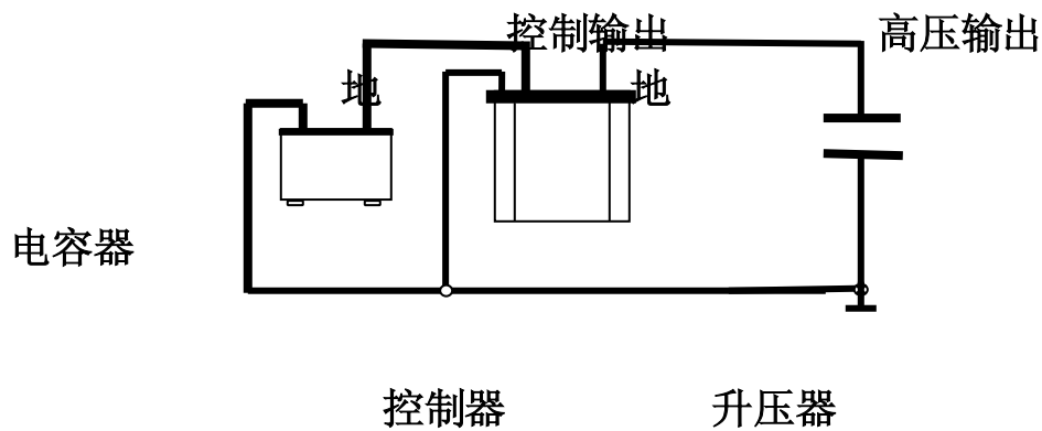
图 19 测量电容器的连线图
