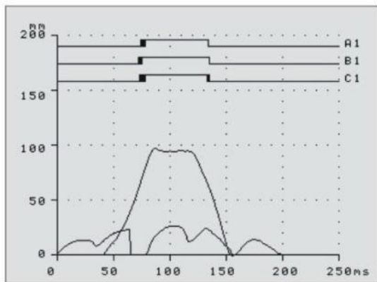
合--分闸测试图形
