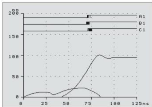
合闸测试图形
