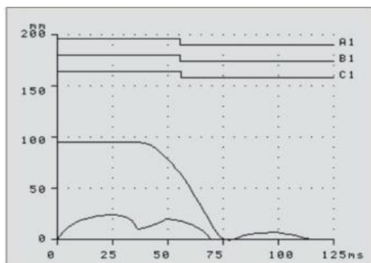
分闸测试图形
